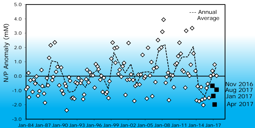
Mixed Layer N-P Anomaly (CalCOFI Std Grid) 198401-201708
