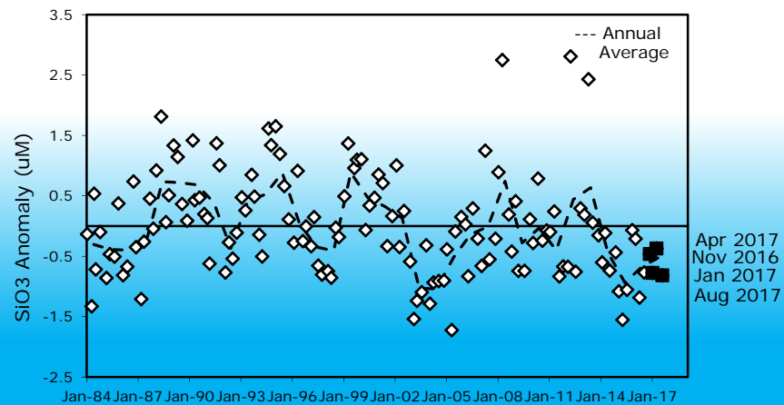
Mixed Layer SiO3 Anomaly (CalCOFI Std Grid) 198401-201708
