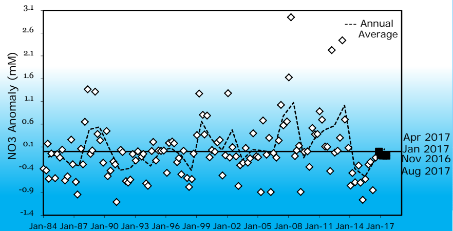
Mixed Layer NO3 Anomaly (CalCOFI Std Grid) 198401-201708
