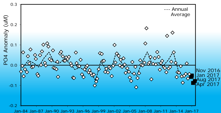
Mixed Layer PO4 Anomaly (CalCOFI Std Grid) 198401-201708
