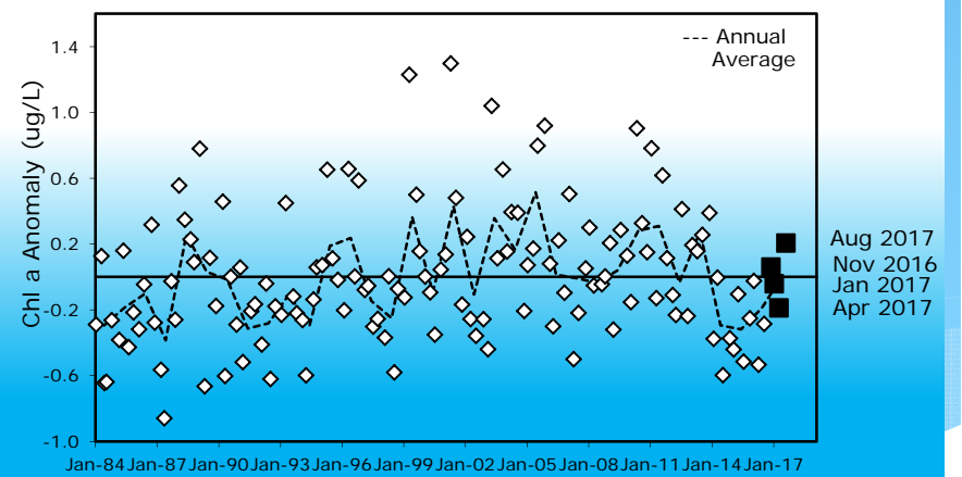
Mixed Layer Chl-a Anomaly (CalCOFI Std Grid) 198401-201708
