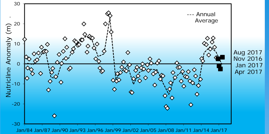
M.L. Nutricline Anomaly (CalCOFI Std Grid) 198401-201708
