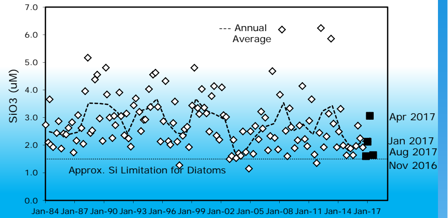
Mixed Layer SiO3 Avg (CalCOFI Std Grid) 198401-201708
