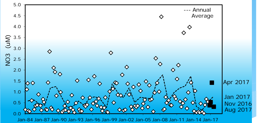
Mixed Layer NO3 Avg (CalCOFI Std Grid) 198401-201708
