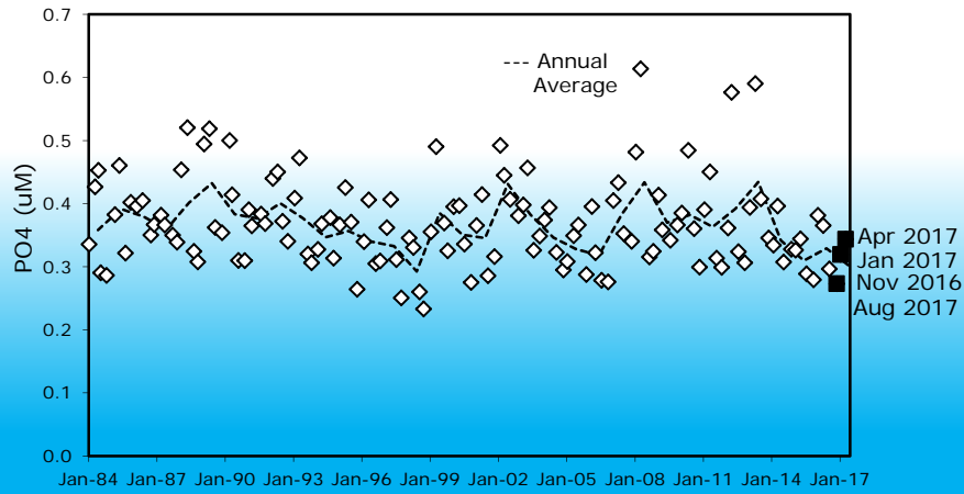
Mixed Layer PO4 Avg (CalCOFI Std Grid) 198401-201708
